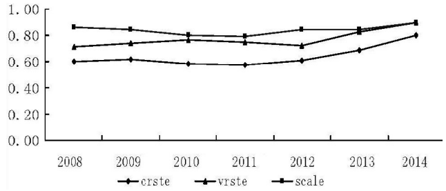
2008~2014年西部地区节能环保产业上市公司融资效率的均值趋势图
